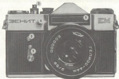
1—рычаг автоспуска; 2—кнопка включения автоспуска; 3—спусковая кнопка с гнездом под тростик; 4—штепсельный разъем для лампы-вспышки; 5—фотоэлемент
