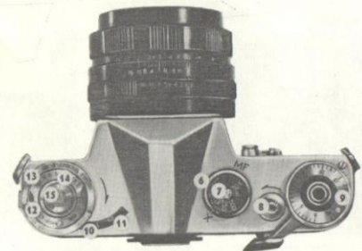
6—диск синхронизации; 7—диск выдержек затвора; 8—штулка отключения затвора; 9—лиimb счетчика кадров; 10—стрелка измерителя экспонометра; 11—стрелка калькулятора; 12—шкала светочувствительности пленки; 13—шкала выдержек калькулятора; 14—шкала диафрагм калькулятора; 15—головка обратной перемотки
