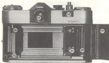
16—поводок кассетной катушки; 17—окуляр видоискателя; 18—рычаг взвода; 19—откидная крышка камеры; 20—приемная катушка; 21—мерный валик; 22—гнездо кассеты
