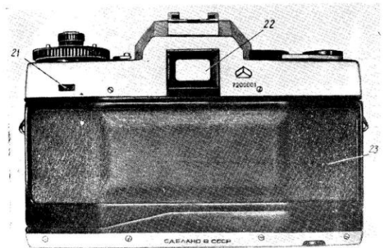
Рис. 4. Вид фотоаппарата сзади:
