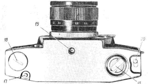
Рис. 3. Вид фотоаппарата снизу:
