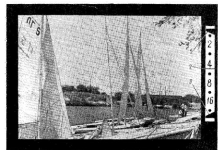
б — фотоаппарат наведен на резкость: 1 — указатель «света мало»; 2 — стрелка гальванометра; 3 — указатель «света много».
