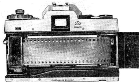
Рис. 9. Заряженный аппарат.
