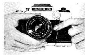
Рис. 17. Смена объектива
